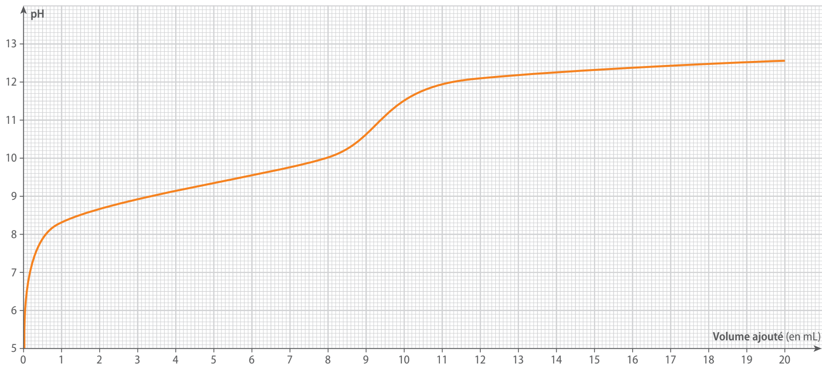
Évolution du pH en fonction du volume ajouté de solution d'hydroxyde de sodium
